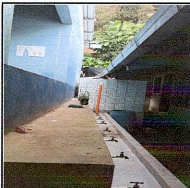
Foto 3: Finalización del tanque de agua y suministro e instalación de bajadas de agua pluviales dentro del mismo.
